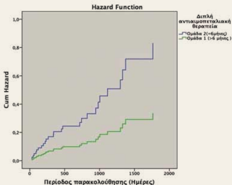
Εικόνα 1. Cox regression- Η μπλέ γραμμή και η πράσινη γραμμή αντιπροσωπεύουν τον στιγμιαίο κίνδυνο θνησιμότητας στην ομάδα 2 και στην ομάδα 1 αντίστοιχα.
